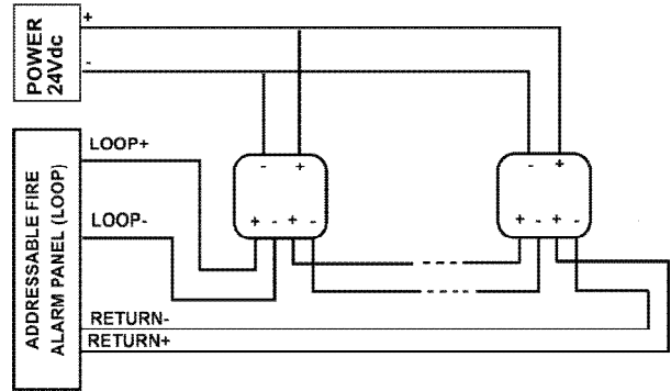
Şekil-2 CO401 Adresli Karbonmonoksit Gaz Dedektör Bağlantısı
